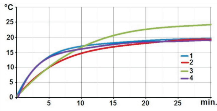
Diagramm des Klemmen-Temperaturanstiegs bei 16A Stromstärke je nach Modell und deren Schutz
